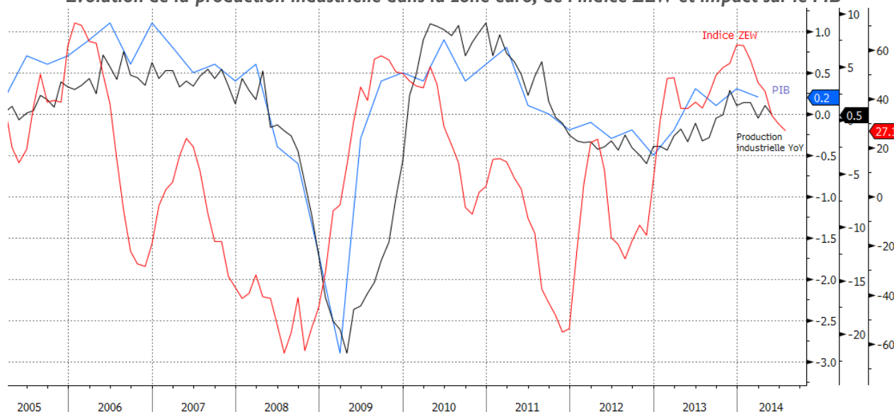
Evolution de la production industrielle dans la zone euro, de l'indice ZEW et impact sur le PIB
